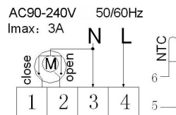
Vízfűtés kapcsolási rajza (ne csatlakoztassa a motoros szelep "close" terminálját)
